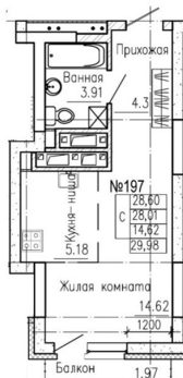
Квартира № 197, этаж 21
