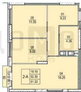
Экспликация помещения
