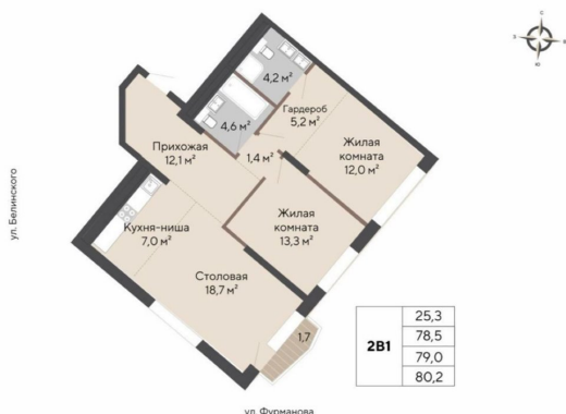
ПРЕДВАРИТЕЛЬНЫЙ ПЛАН КВАРТИРЫ (этаж 18, секция 1.2)
