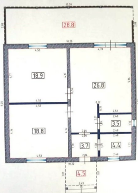
ПЛАН ЗДАНИЯ
